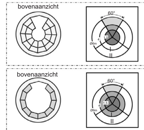
Fig.6: detectieveld
