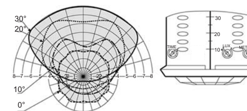
Fig.6: detectieveld
