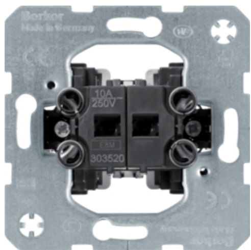
Jaloezieschakelaar 1-polig
