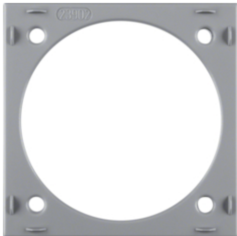
Opbouw-afstandsring, berker Integro, grijs
