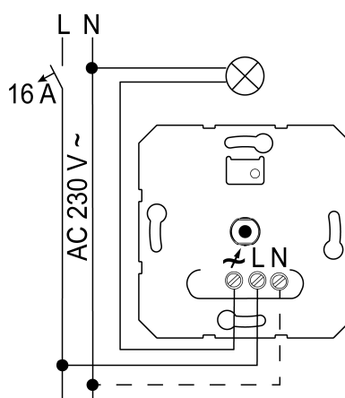
Afbeelding 3: Aansluitschema
