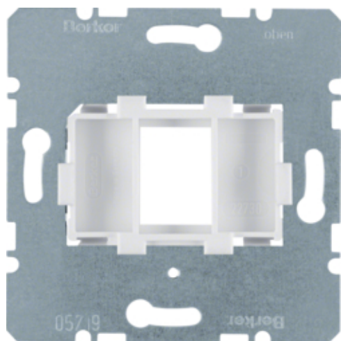
Draagplaat modulaire jacks, 1-voudig, witte houder (14,9 x 20,7 mm)
