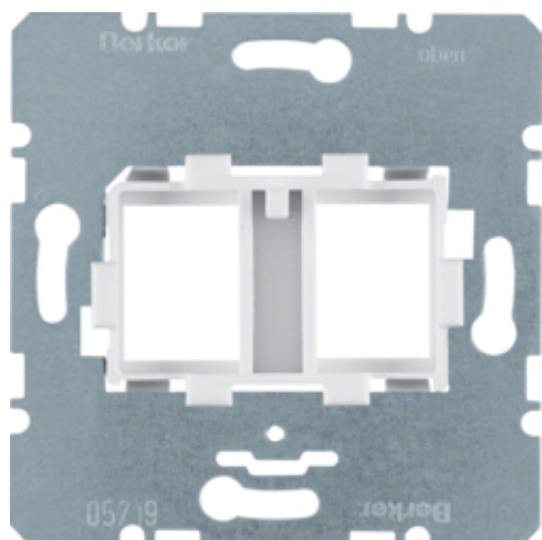
Draagplaat modulaire jacks, 2-voudig, witte houder (14,9 x 20,7 mm)
