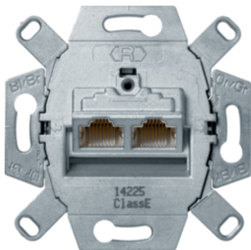
RJ-datacontactdoos 2-voudig, cat. 6, 45° -uitgang
