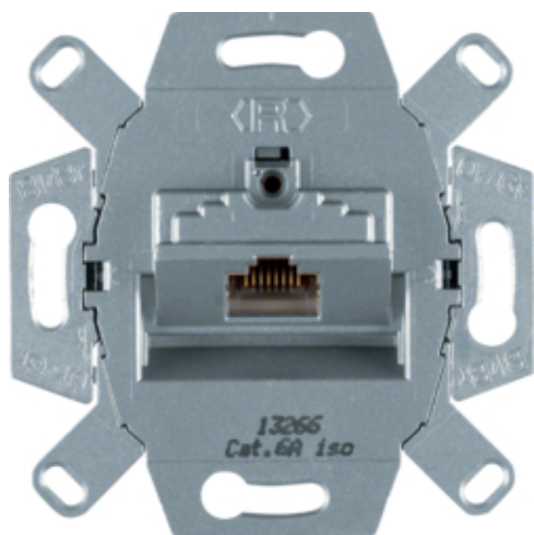
RJ-datacontactdoos 1-voudig, cat. 6A, 45° -uitgang
