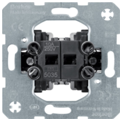
Serie-impulsdrukker, 2 maakcontacten, gedeelde ingang
