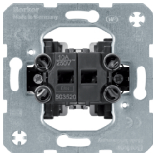
Jaloezie-impulsdrukker, 1-polig
