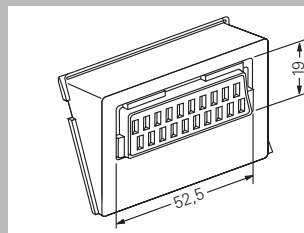
Inzetstuk met Scart/Euro-AV-bus 0093 00
