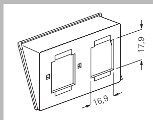
Inzetstuk voor Modular Jack/Western Techniek AMP/Radiall, 1voudig 0052 00
