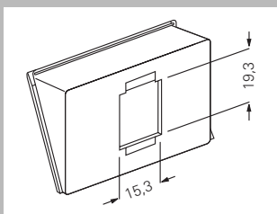
Inzetstuk voor Modular Jack/Western Techniek AMP/Radiall, 1voudig 0052 00
