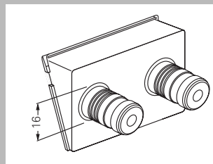
Inzetstuk met geïntegreerde High-End luidspreker-connector WBT (+/-) 0091 00
