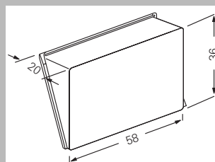
Blind inzetstuk 0048 00
