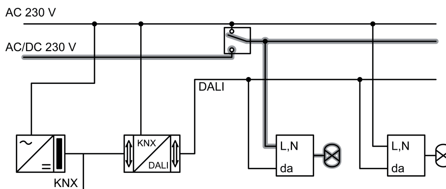
Afbeelding 3: Noodverlichting door centrale beveiligingsvoeding van stroom voorzien
