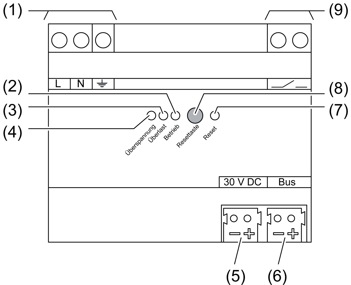
Afbeelding 2: Voeding 1280 mA – aanzicht
