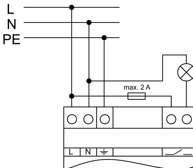
Afbeelding 5: Toepassingsvoorbeeld – meldlamp voor optische bedrijfsindicatie
