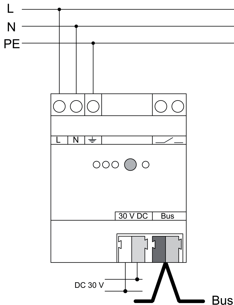
Afbeelding 3: Aansluitvoorbeeld – netspanning en buslijn
