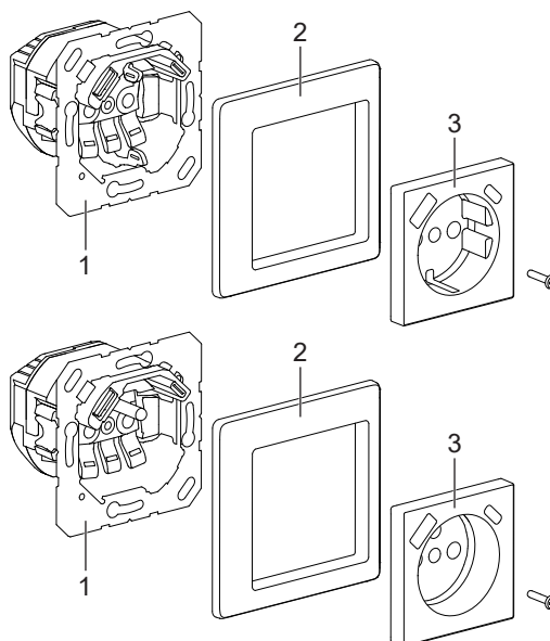
Afb. 1: Constructie apparaat
