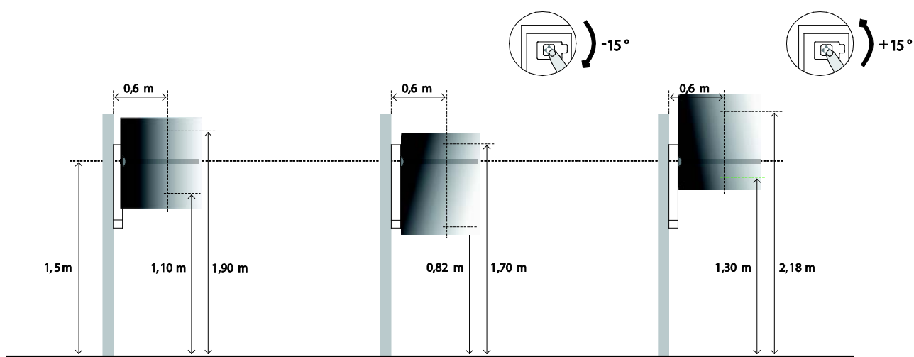
Afb. 10: Detectiehoek verticaal
