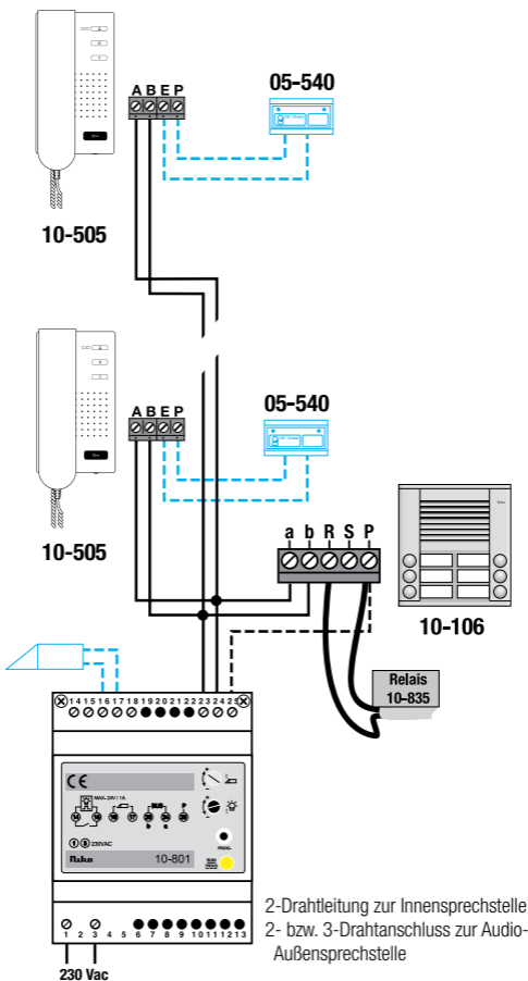
Abb. 4: vollständiger Anschlussplan
