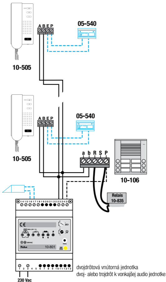
Obr. 4: kompletná schéma zapojenia
