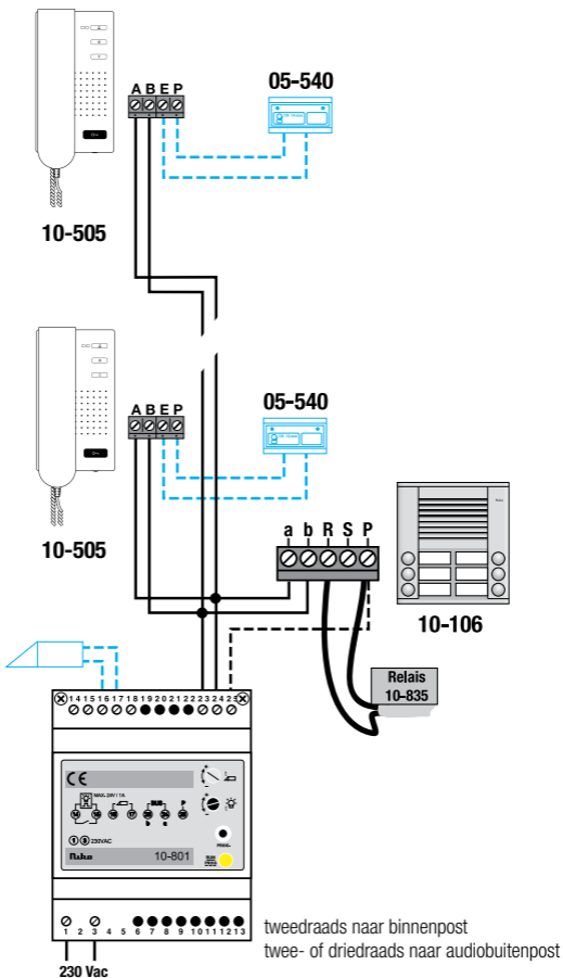
Fig. 4: compleet aansluitschema
