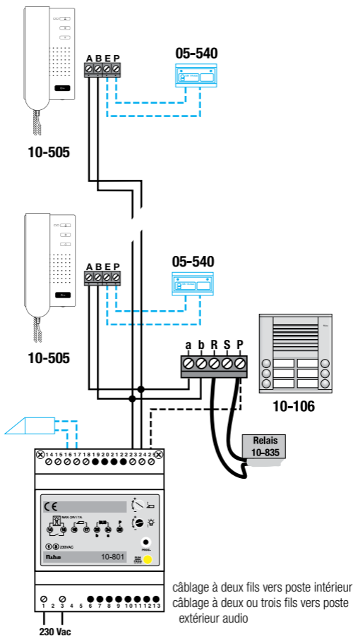
Fig. 4 : schéma de raccordement complet
