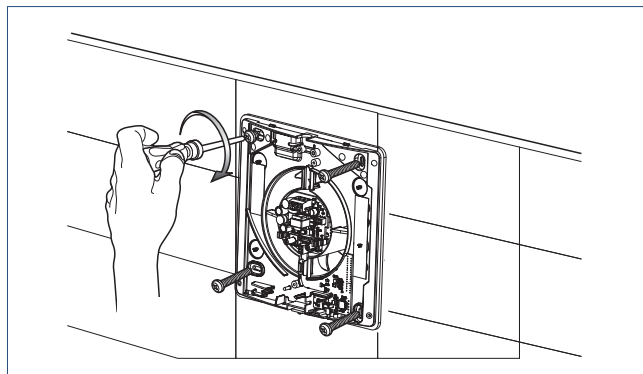
i) Plaats de ventilator (met de meegeleverde witte foam tussen de wand en de ventilator om trillingen en luchtlek te verminderen) en schroef deze in de muur of plafond.
